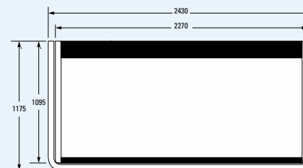
Tobago 2270 pianta testata
